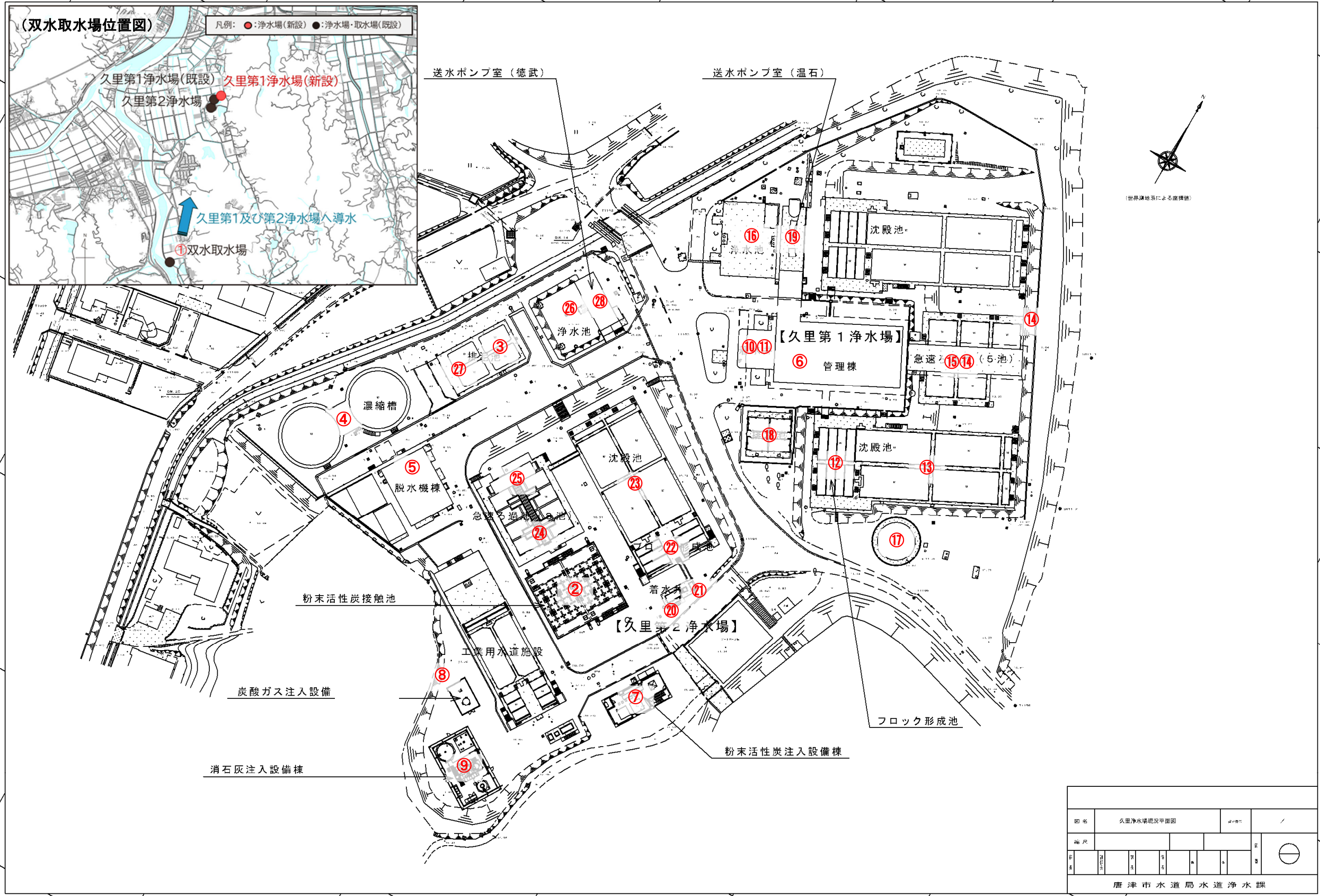
(別紙2: 既設久里第1浄水場及び既設久里第2浄水場 図面)
