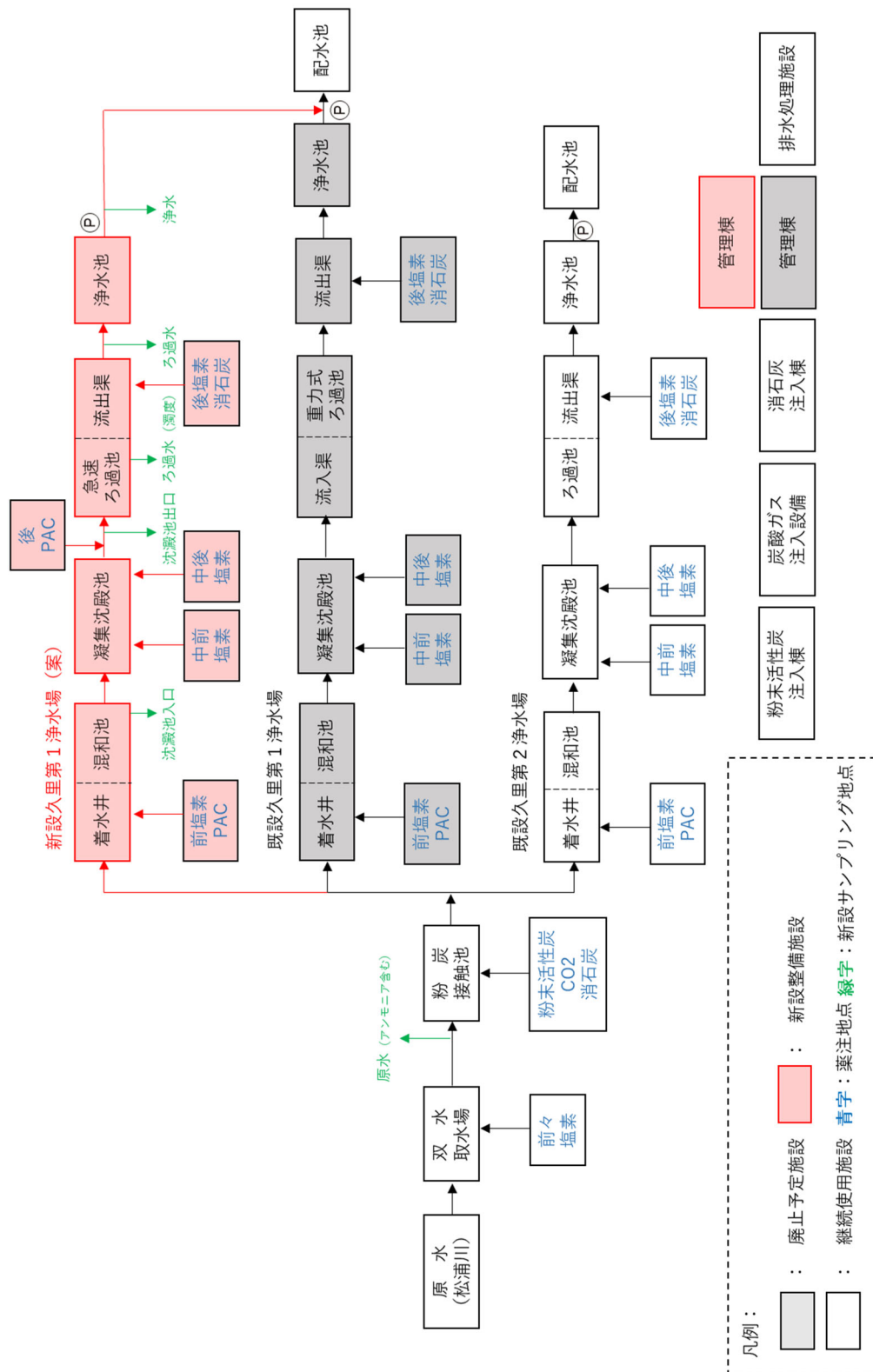
図2-2 更新前後の施設フロー(案)
