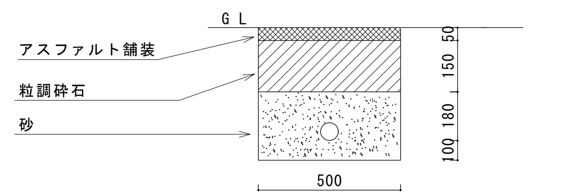
給水管埋設要領図 アスファルト部
