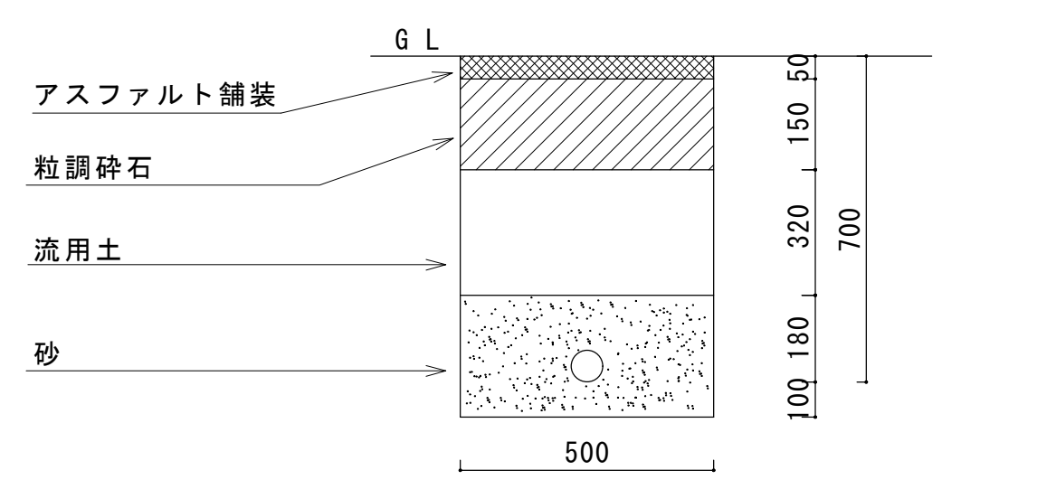
ポンプ圧送管埋設要領図 アスファルト部
