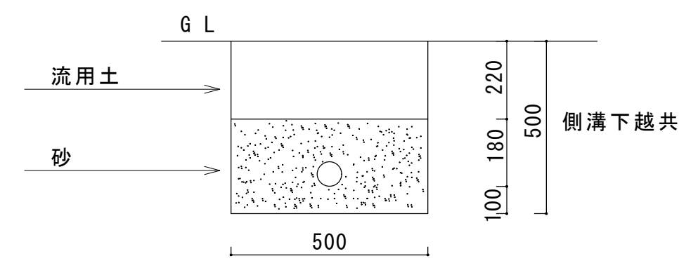
ポンプ圧送管埋設要領図 植栽部
