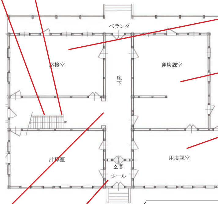
1階平面図
