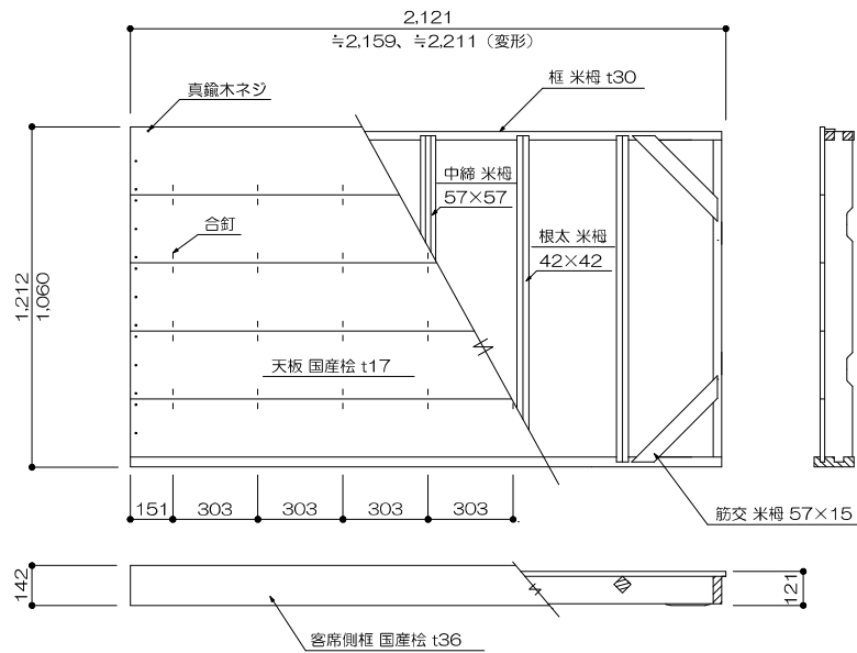
2~5 花道所作台 1/20
