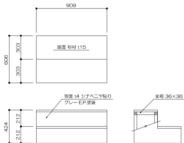
31 ヒナ段用階段 1/20
