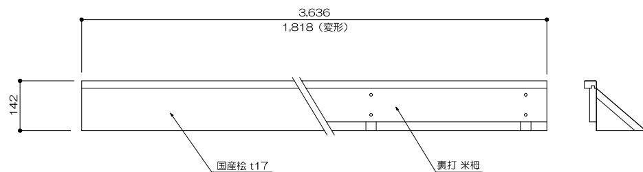
9、10 化粧框 1/10
