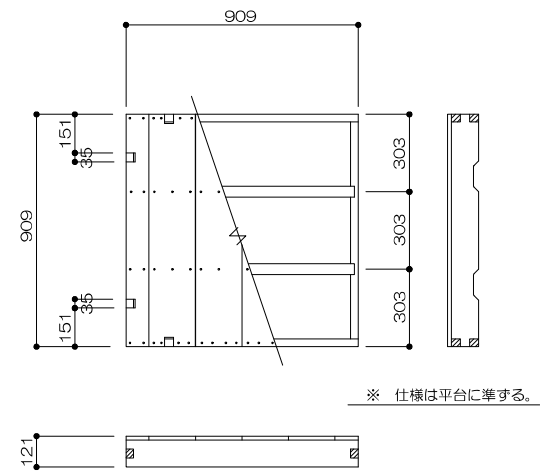
20 平 台 1/20
