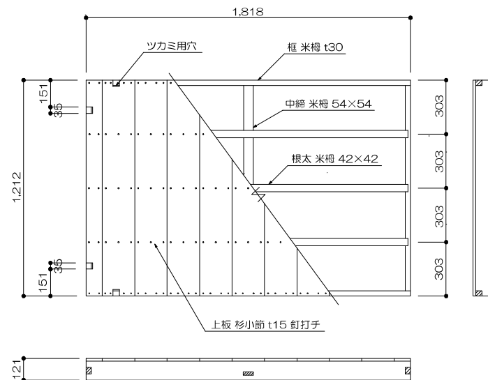
16 平 台 1/20
