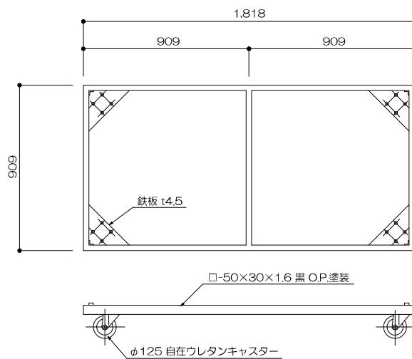
45 平台運搬車 1/20
