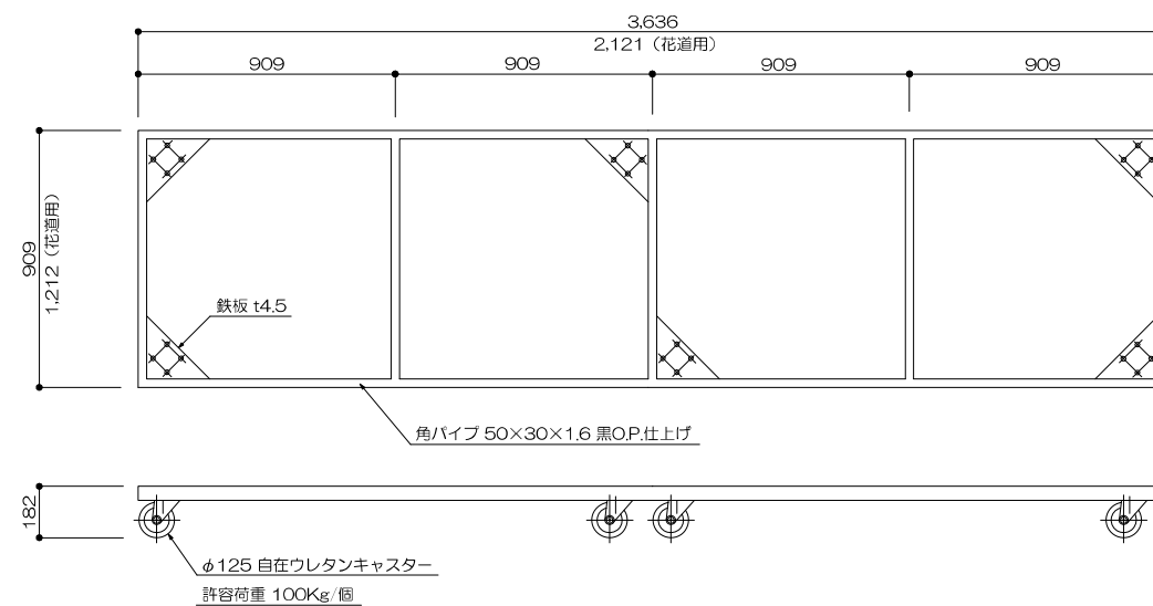
11、12 所作台運搬車 1/20
