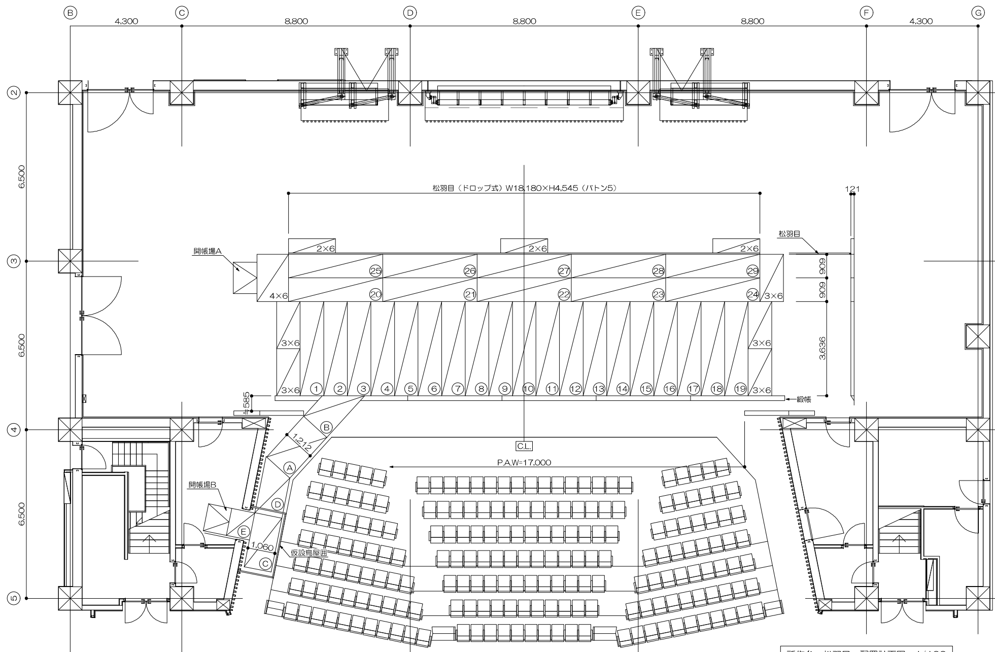
所作台・松羽目 配置計画図 1/100
