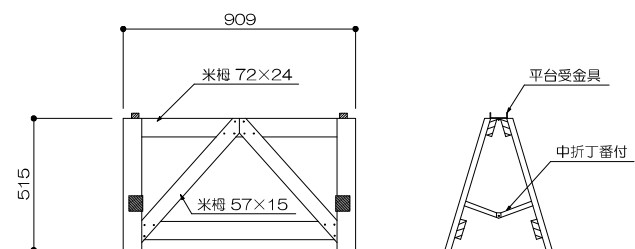
26 開き足 (中足) 1/20
