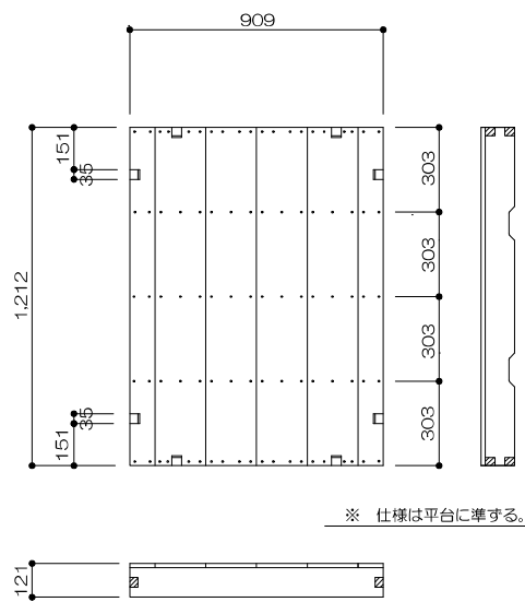
19 平 台 1/20
