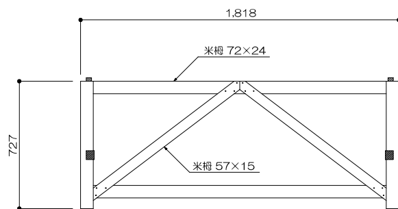
21 開き足 (高足) 1/20
