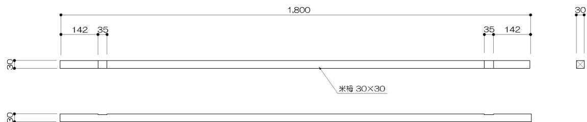
48 ツカミ金具 1/2
