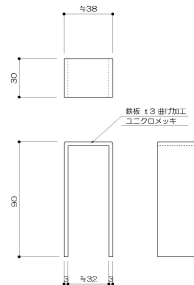
47 滑り止め木用金具 1/2
