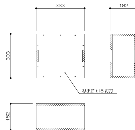
28 箱 足 1/10
