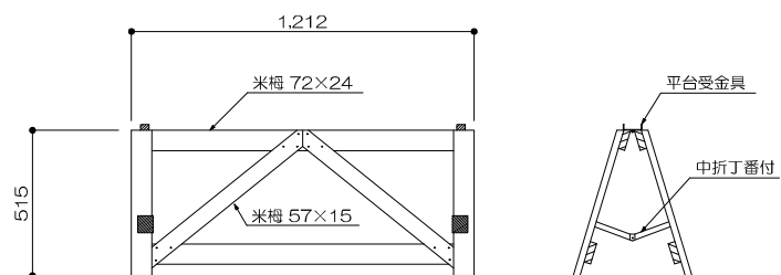
25 開き足 (中足) 1/20
