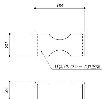
48 ツカミ金具 1/2
