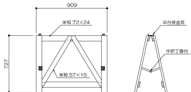
23 開き足 (高足) 1/20
