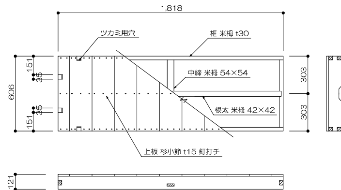
18 平 台 1/20
