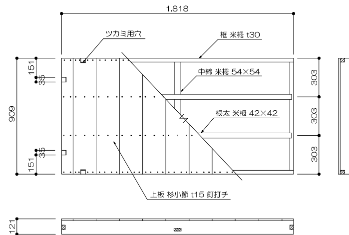
17 平 台 1/20
