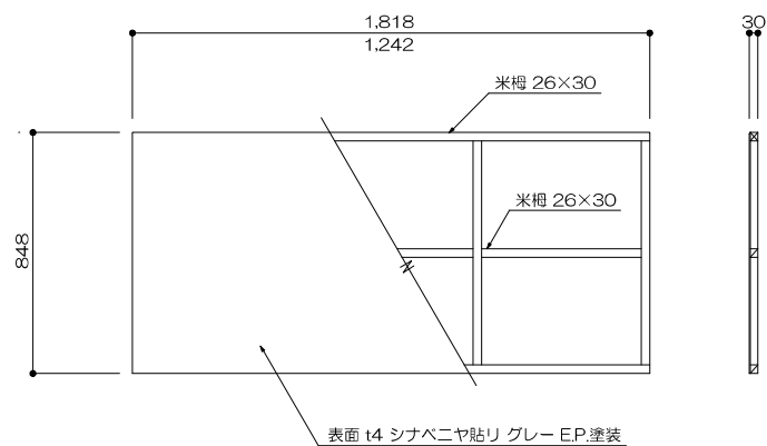
33、38 蹴込パネル 1/20
