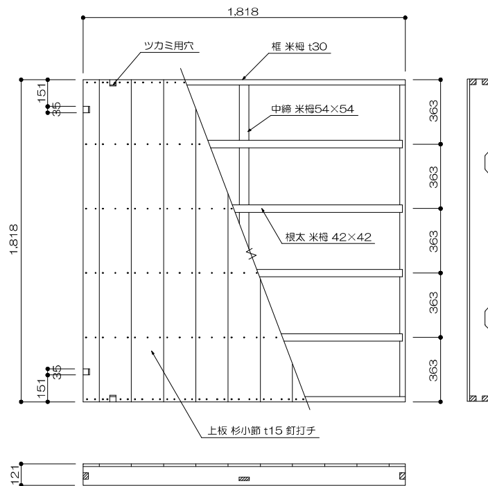
15 平 台 1/20
