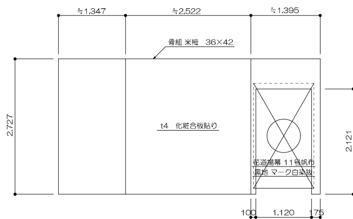
13 仮設鳥屋囲 1/50
