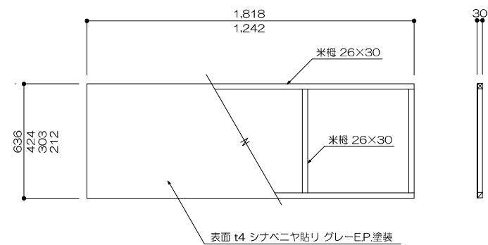
34~37、39~42 蹴込パネル 1/20
