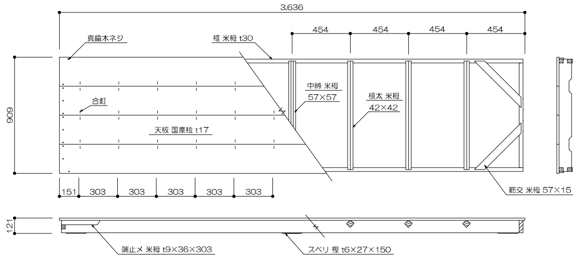
1 所作台 1/20
