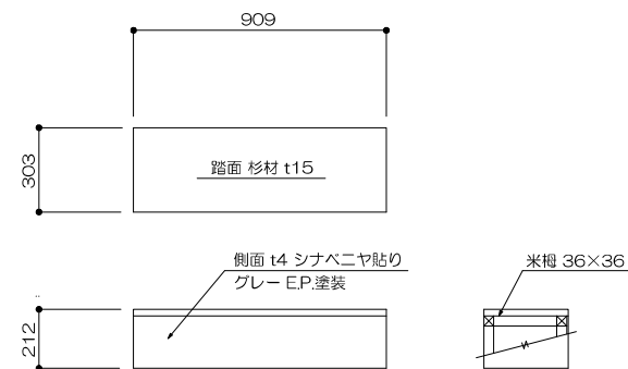
32 ヒナ段用階段 1/20
