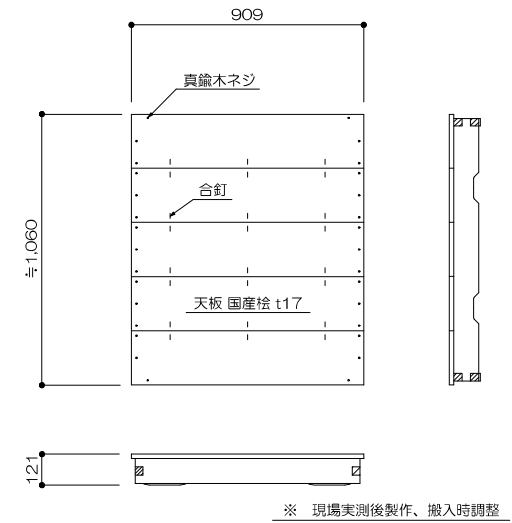
6 花道所作台 1/20
