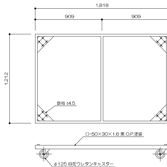
46 滑り止め木 1/10
