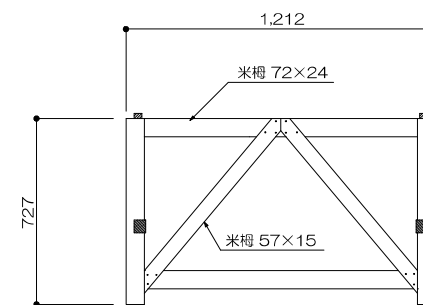
22 開き足 (高足) 1/20
