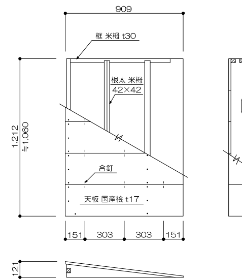
7、8 開帳場 1/20
