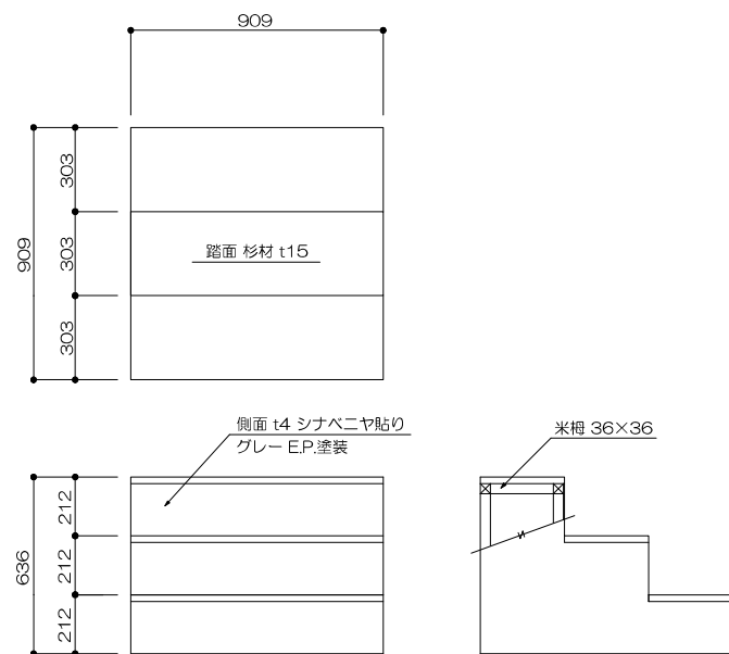
30 ヒナ段用階段 1/20
