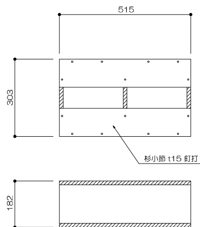
27 箱 足 1/10
