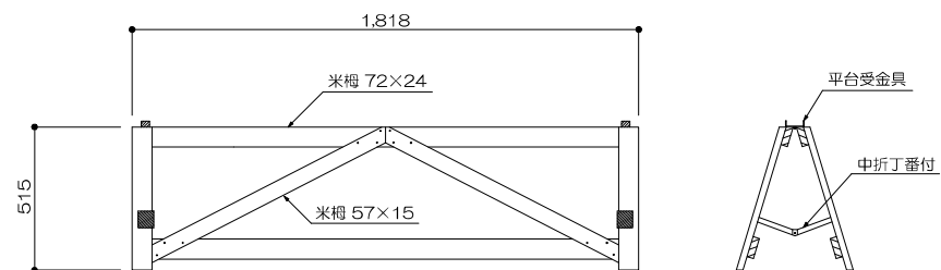
24 開き足 (中足) 1/20
