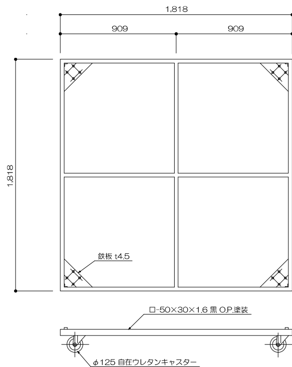
43 平台運搬車 1/20
