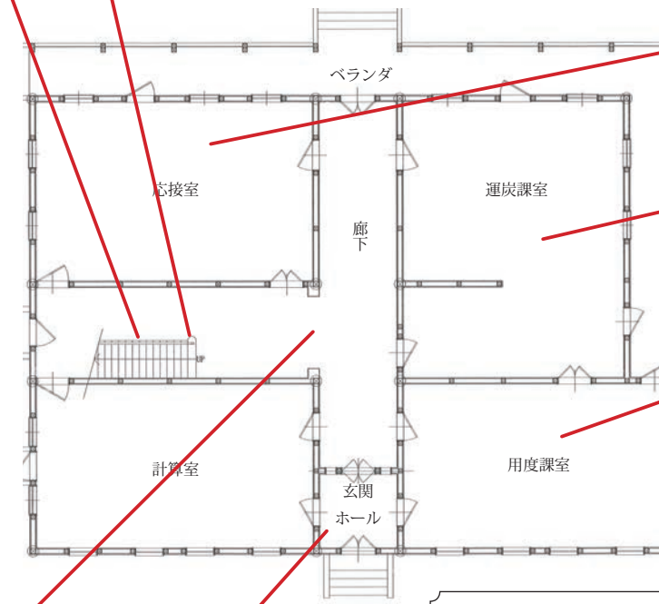
1階平面図
